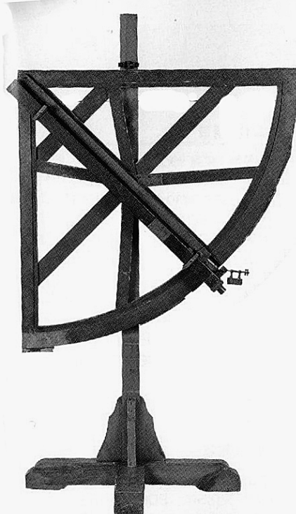
中象限儀模型 恒星の高度を測るために使われた。天体観測のメインの機器である。四半円部は伊能隊が利用した実物だが支柱は仮柱である。
